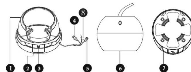
Câmera dome.
